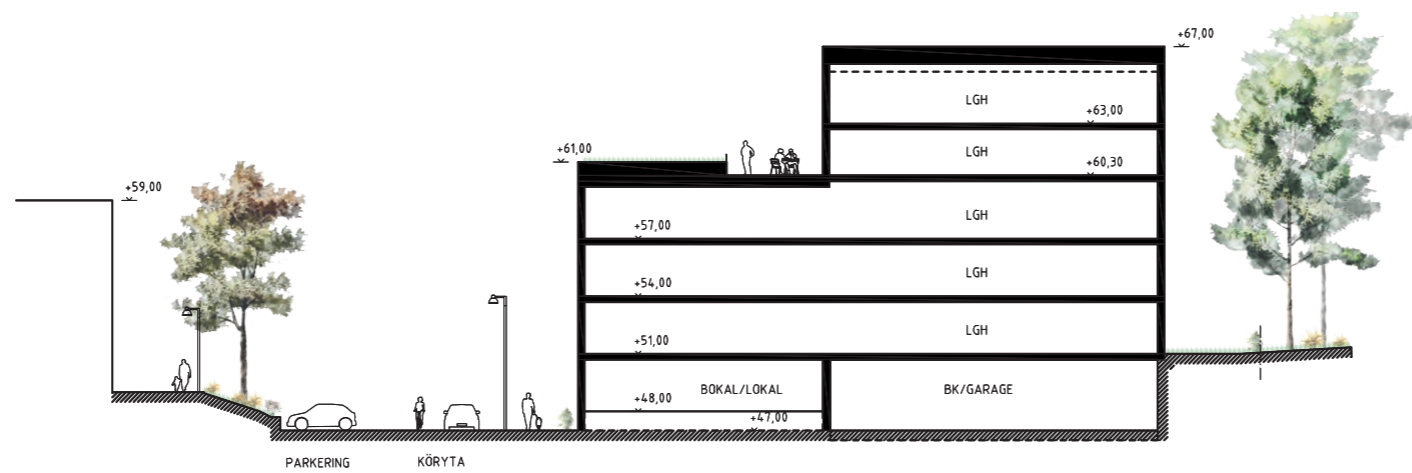
SEKTION A-A
