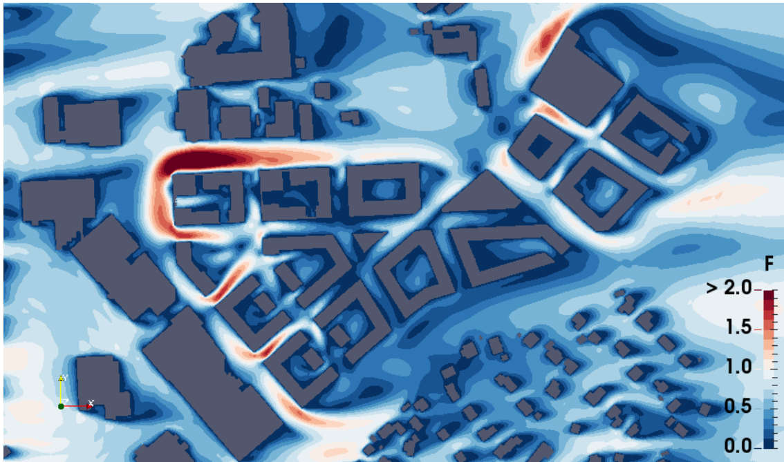
Figur 10: Vindens förstärkning ( F ) vid västlig vind ( 270^\circ ) på fotgängarnivå två meter ovan mark. Faktorn anger förstärkning relativt bakgrundsvinden på samma nivå.
